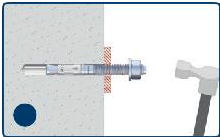
安装锚栓
