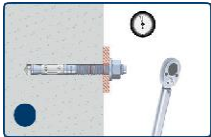
施加扭矩
